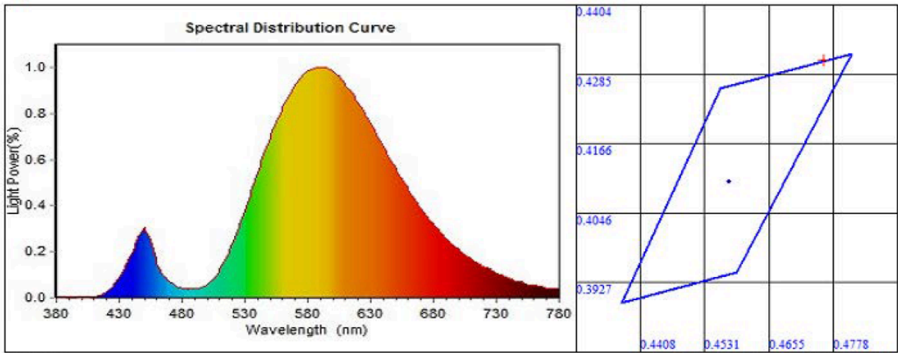
光谱分布
